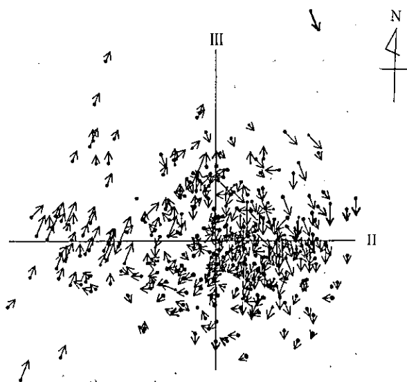
図2.21 主成分パターンの各日の重みと風向風速との関係
