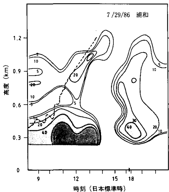
図2.5 二酸化窒素高度分布の時間変化 図中の破線は混合層高度。
