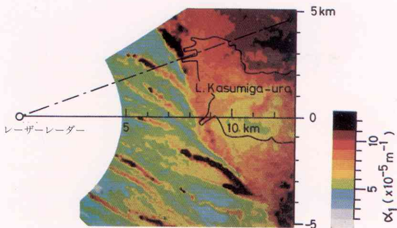
口絵写真2 レーザーレーダーによる PPI 観測から得られたエアロゾル濃度水平分布 (本文 7, 20, 22 頁参照) 消散係数 \alpha_1 (単位: \text{m}^{-1} ) の形で得られたエアロゾル濃度は、10 レベルでカラー表示されている。 (空気分子による消散係数 \alpha_2 は、15°C, 1 気圧で 1.33 \times 10^{-6} \text{ m}^{-1} である)
