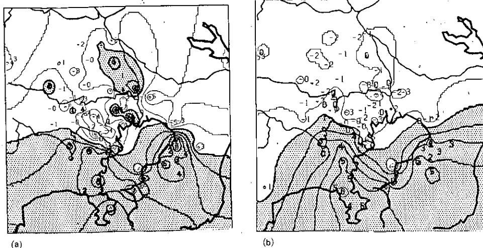
図2.20 二酸化硫黄の第2主成分パターン（因子負荷量）
